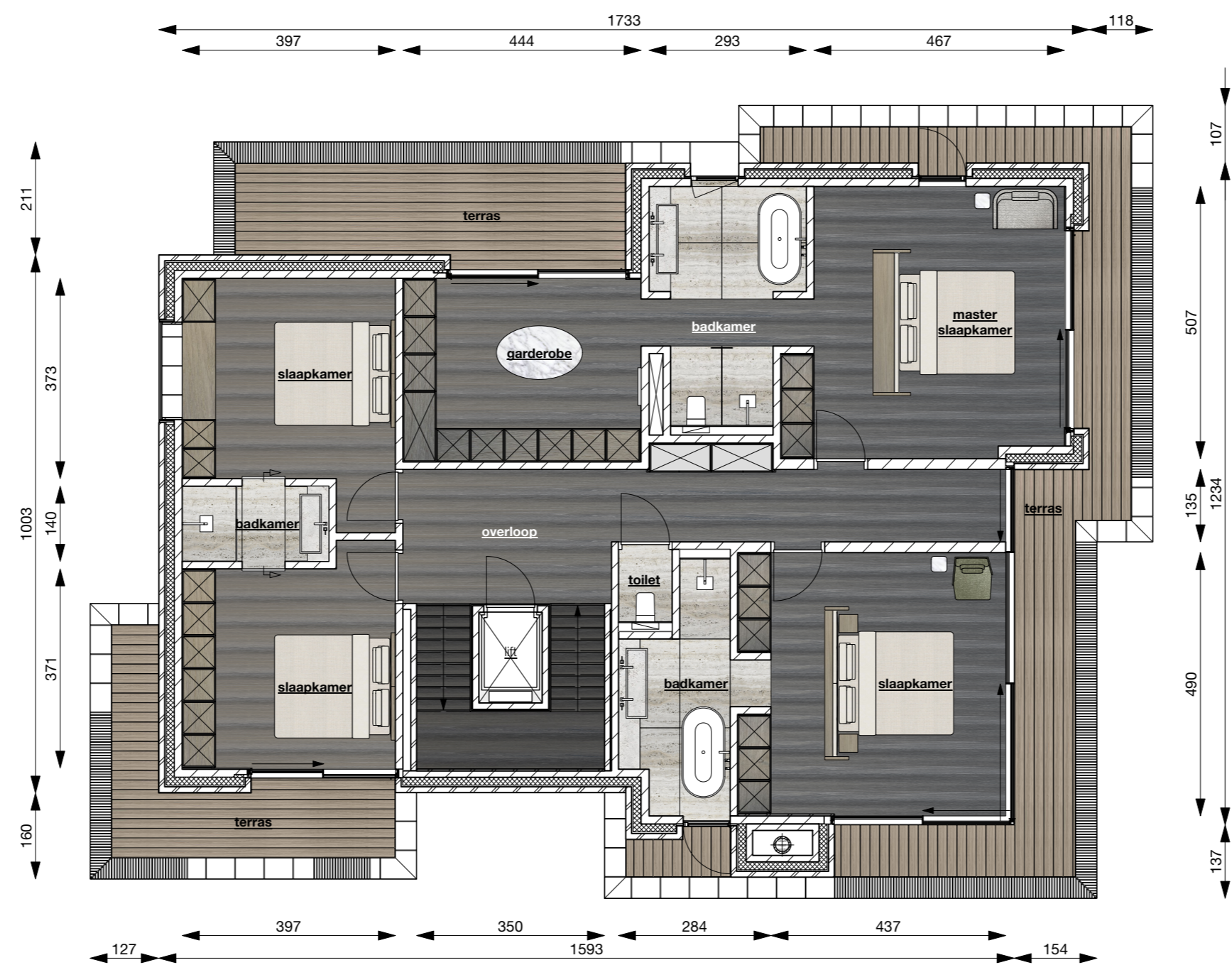
PLATTEGROND 1e VERDIEPING
